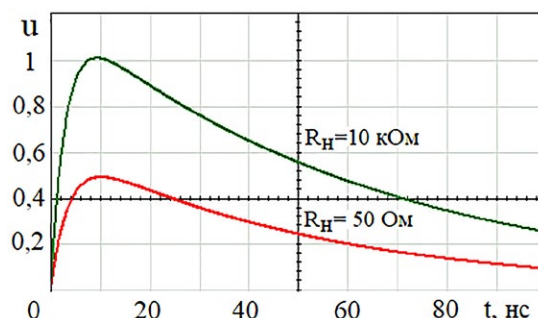
Рис. 2. Изменение напряжения u на выходе модели испытательного генератора по IEC 61000-4-4 при нагрузке R_H=R4 с сопротивлением 50 Ом и 10 кОм.
